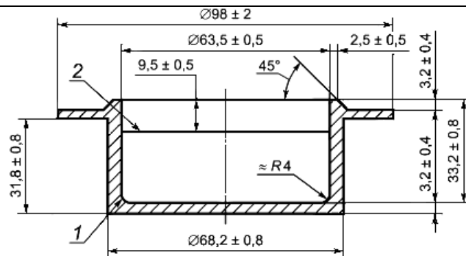
1 - открытый тигель; 2 - уровень заполнения тигля битумом
