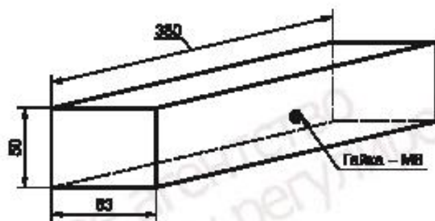
Рисунок 2 — Расположение гайки
