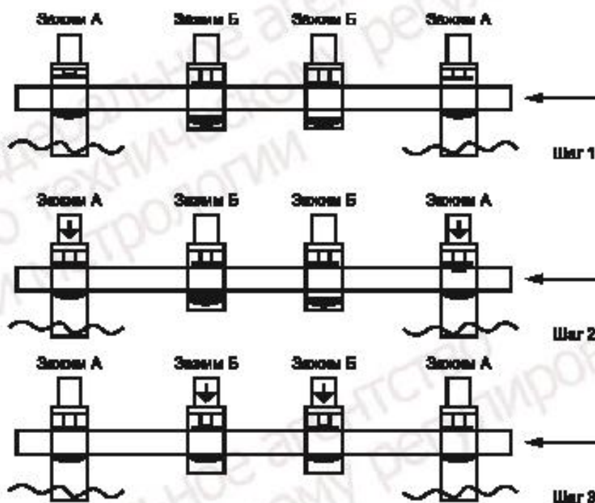
Рисунок 3 — Процедура размещения образца в зажимах
