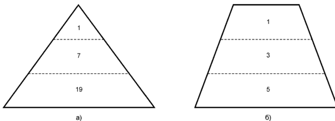
Рисунок 1 - Схема отбора точечных проб из штабелей конусообразной (а) и призматической (б) форм
