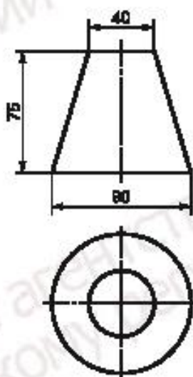
Рисунок 1 — Металлическая форма
