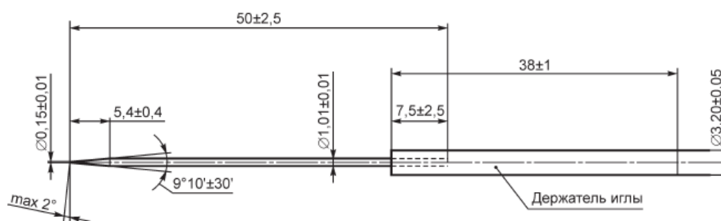
Рисунок 1 - Пенетрационная игла
