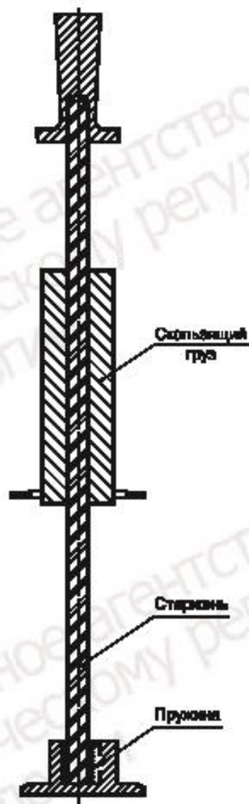
Рисунок 2 — Схема уплотнительного молота
