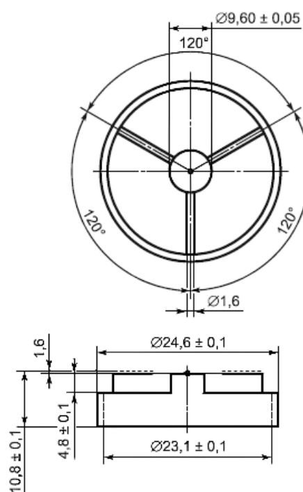
Рисунок А.4 - Нижняя пластинка
