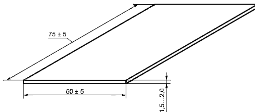
Рисунок А.6 - Заливающая полированная пластинка
